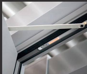
Im Türblatt verdeckter Türschließer – optional
